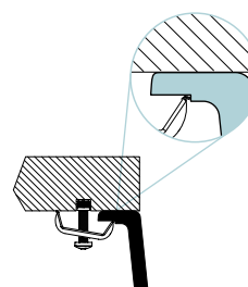
Spodní uložení Instalace s příchýtkami
