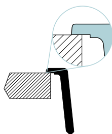
Horní uložení Instalace bez příchytěk
