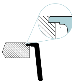
Uložení do roviny Instalace bez příchytěk
